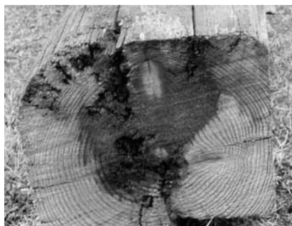
Gennemskåret rådden krøjbjælke. Foto: Asger Mansted
